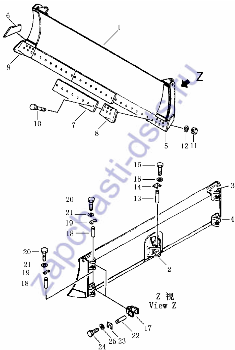
第 705 图 角 铲 FIG.705 ANGLE BLADE
