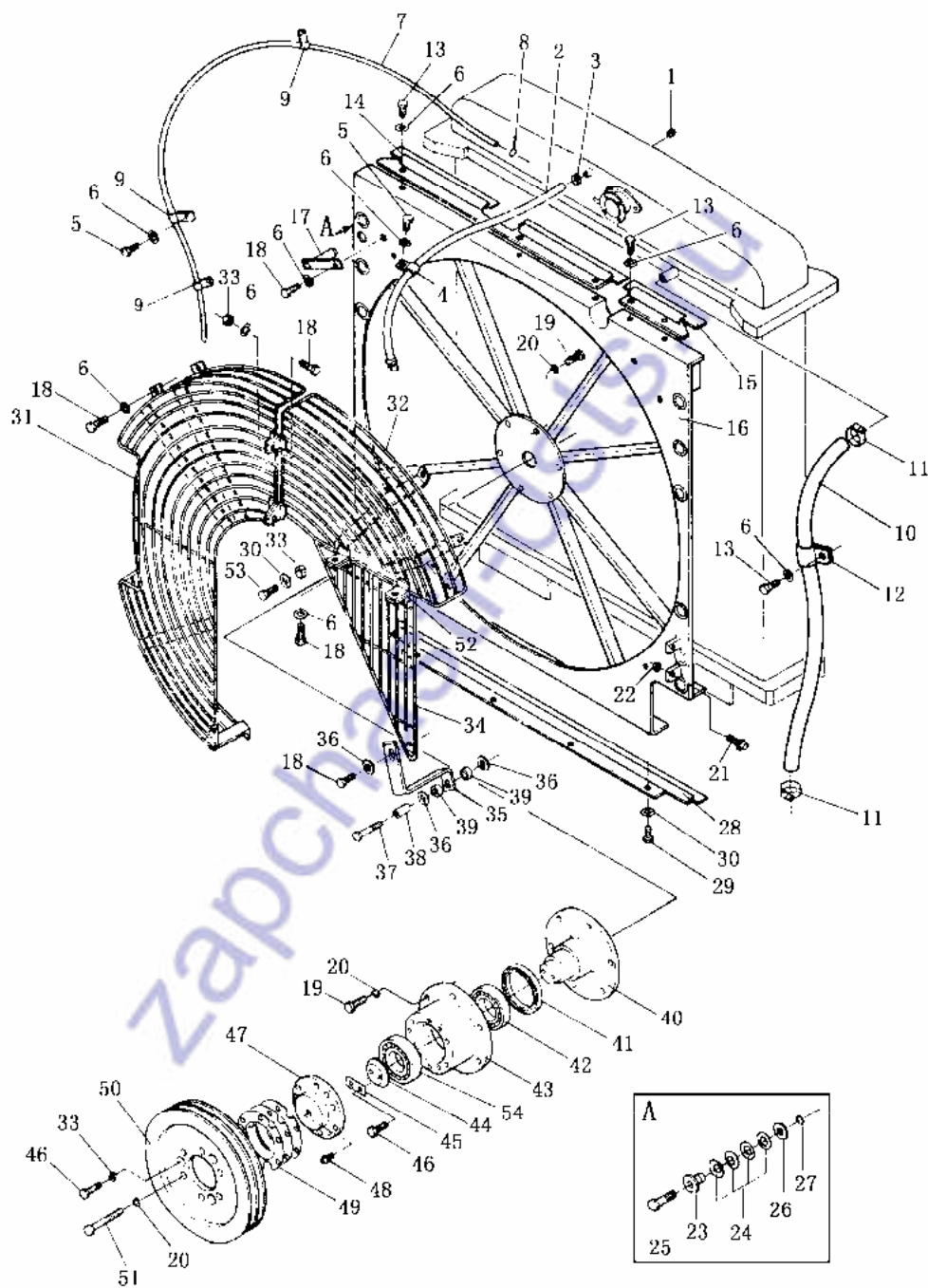
第 109 图 散热器管路及护风罩 FIG. 109 RADIATOR PIPING AND WIND BREAK
